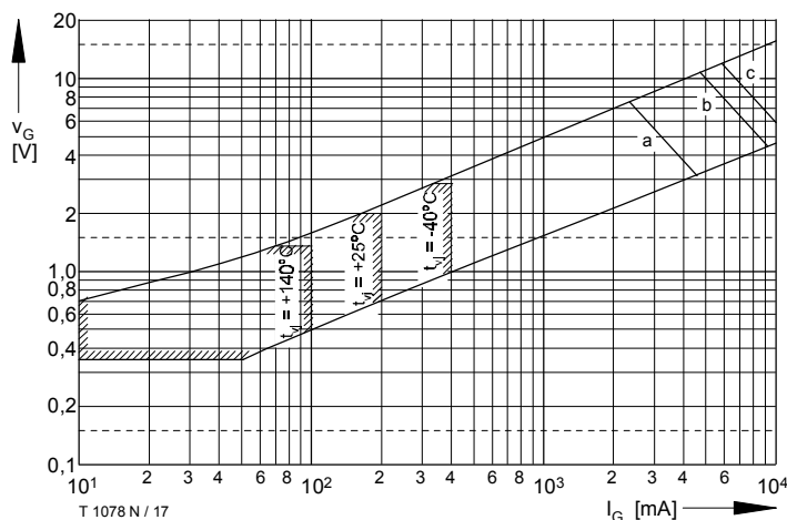
Bild / Fig. 17 Steuercharakteristik mit Zündbereichen / Gate characteristic with triggering areas V_G = f(I_G) , V_D = 6\text{V} Parameter: a b c Steuerimpulsdauer / trigger pulse duration t_G [ms] 10 1 0,5 Höchstzulässige Spitzensteuerverlustleistung / Max. rated peak gate power dissipation P_{GM} [W] 20 40 60
