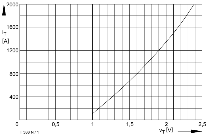
T 388 N / 1 Bild / Fig. 1 Grenzdurchlaßkennlinie / Limiting on-state characteristic i_T = f(v_T) , t_{vj} = t_{vj \text{ max}}
