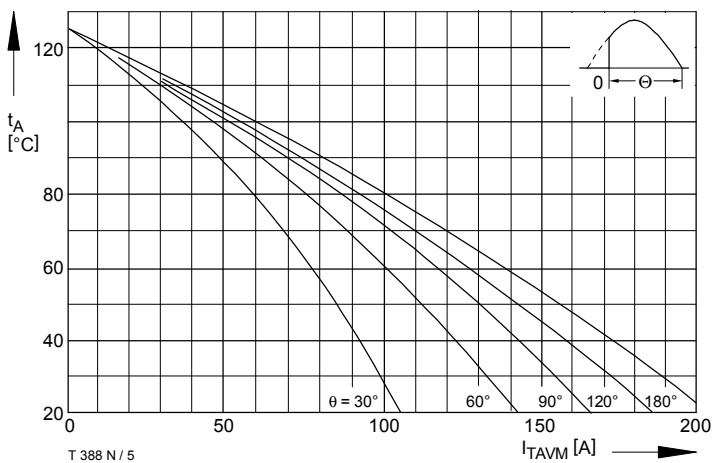
T 388 N / 5 Bild / Fig. 5 Höchstzulässige Kühlmitteltemperatur / Max. allowable cooling medium temperature t_A = f(I_{TAVM}) Luftselbstkühlung / Natural air-cooling Kühlkörper / Heatsink: K0.36S Parameter: Stromflußwinkel / Current conduction angle \theta
