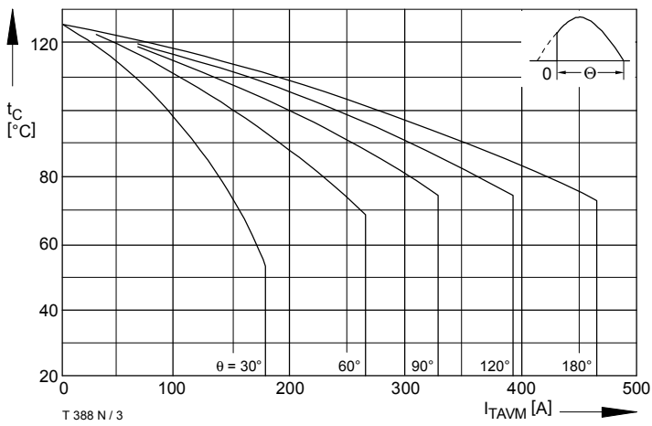
T 388 N / 3 Bild / Fig. 3 Höchstzulässige Gehäusetemperatur / Max. allowable case temperature t_C = f(I_{TAVM}) Beidseitige Kühlung / Two-sided cooling Parameter: Stromflußwinkel / Current conduction angle \theta
