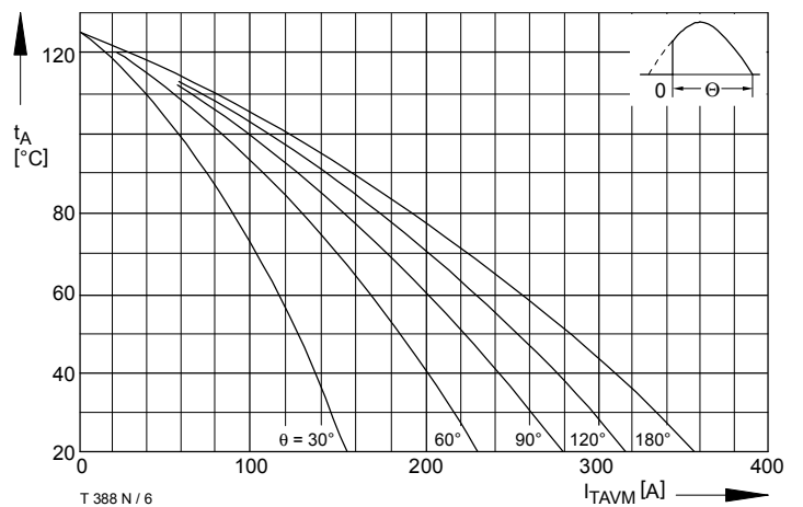
T 388 N / 6 Bild / Fig. 6 Höchstzulässige Kühlmitteltemperatur / Max. allowable cooling medium temperature t_A = f(I_{TAVM}) Verstärkte Luftkühlung / Forced air cooling Kühlkörper / Heatsink: K0.12F, V_L = 50 \text{ l/s} Parameter: Stromflußwinkel / Current conduction angle \theta
