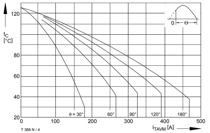
T 388 N / 4 Bild / Fig. 4 Höchstzulässige Gehäusetemperatur / Max. allowable case temperature t_C = f(I_{TAVM}) Anodenseitige Kühlung / Anode-sided cooling Parameter: Stromflußwinkel / Current conduction angle \theta
