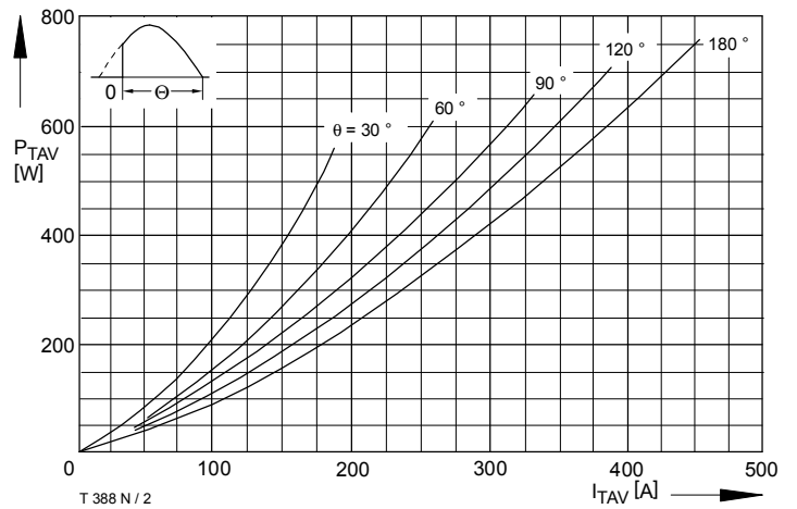
T 388 N / 2 Bild / Fig. 2 Durchlaßverlustleistung / On-state power loss P_{TAV} = f(I_{TAV}) Parameter: Stromflußwinkel / Current conduction angle \theta
